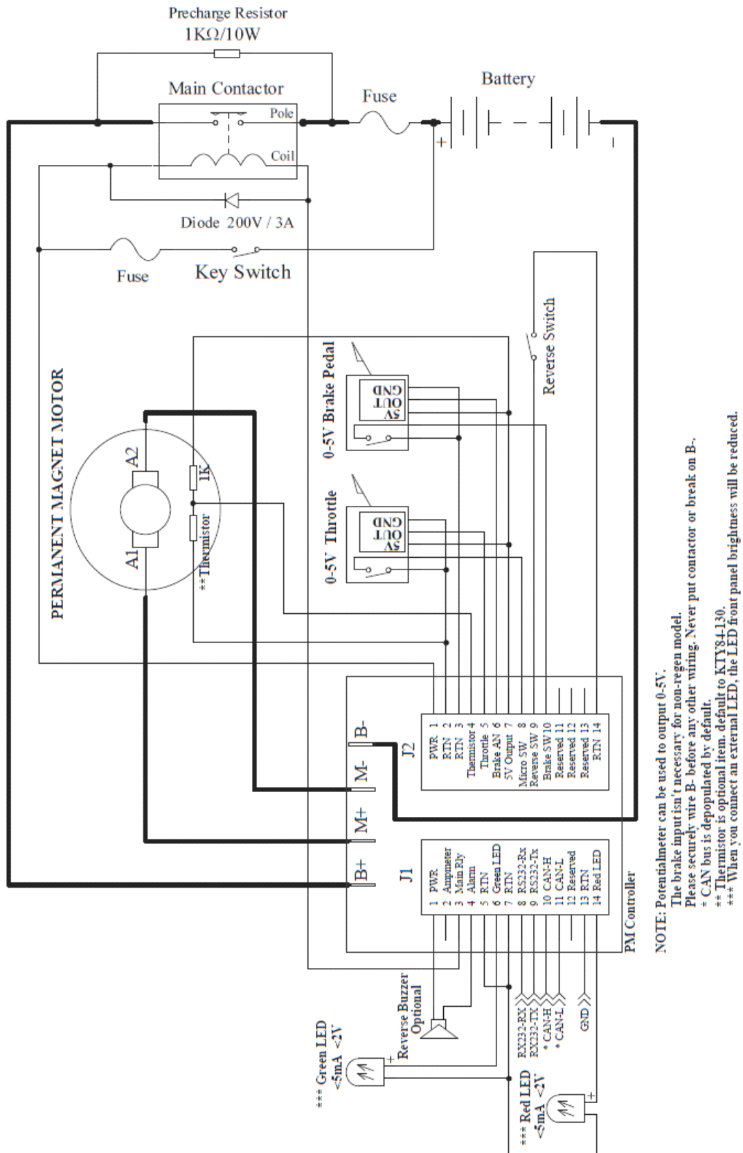
图 4：凯利 PM 全桥永磁电机控制器标准接线图
