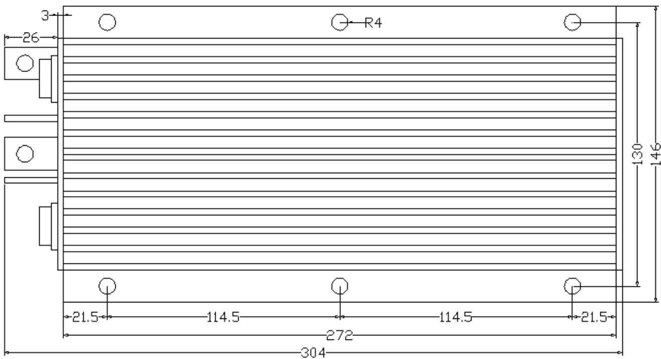
高度：62 毫米 图 2:PM-B 型号的安装孔尺寸(单位:毫米)
