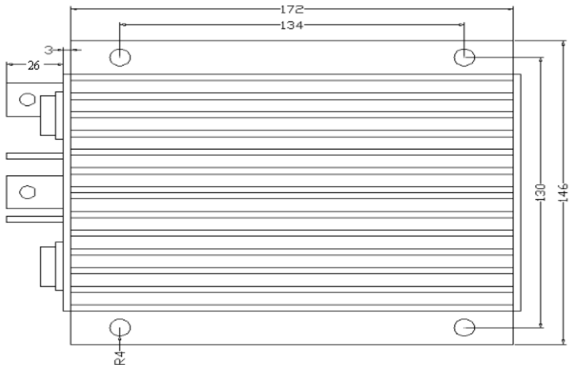
高度：62 毫米 图 1:安装孔尺寸(单位:毫米)
