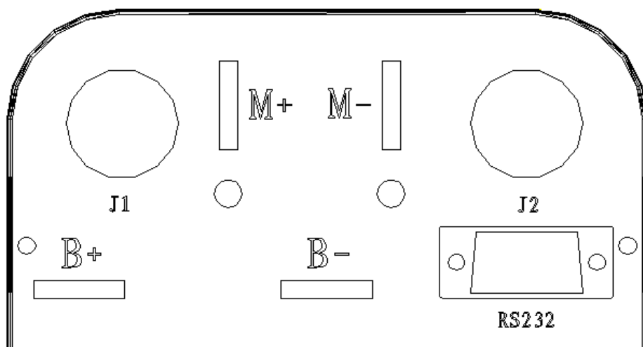
图 3: PM 电机控制器前面板
