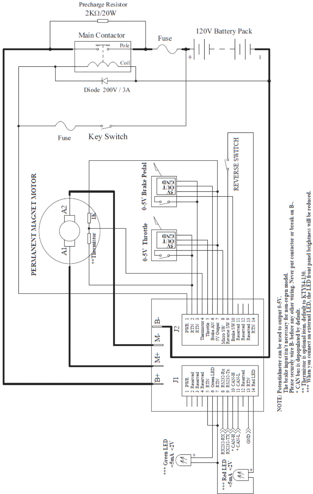
图 5: 120V PM 全桥永磁电机控制器标准接线图
